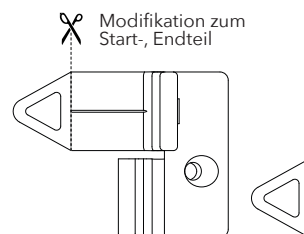
Teilsicht-Verschraubung bei End- und Startdiele
