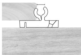
Verbinder-Vorspannung
